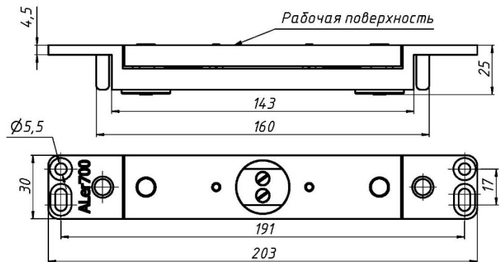
Рисунок 4 - Якорная часть
