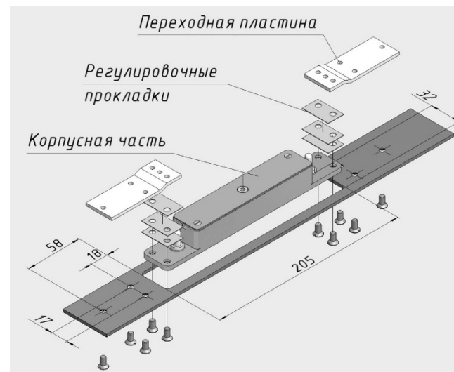
Рисунок 6 - Установка корпуса замка в металлическую коробку
