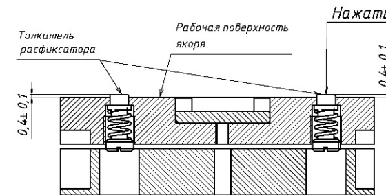
Рисунок 10 – Проверка расфиксатора
