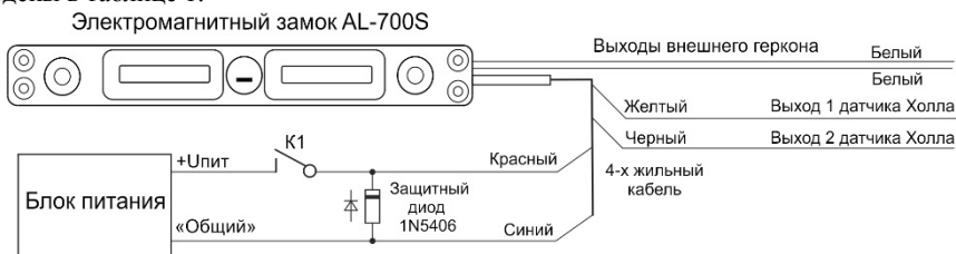
Рисунок 9 - Схема подключения
