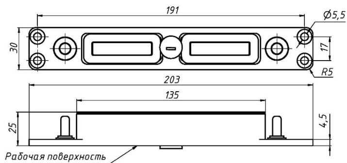
Рисунок 5 - Корпусная часть
